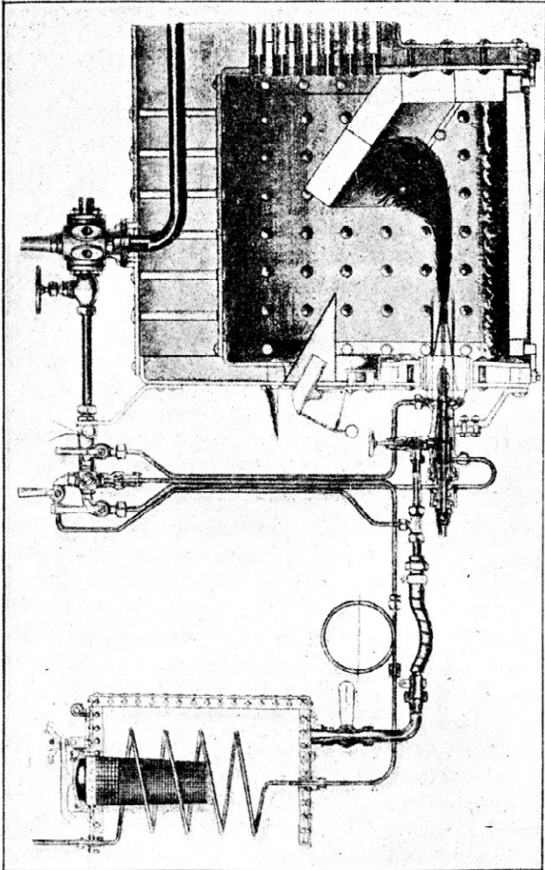
Фиг. 57. Оборудование паровоза, отапливаемого нефтью.
