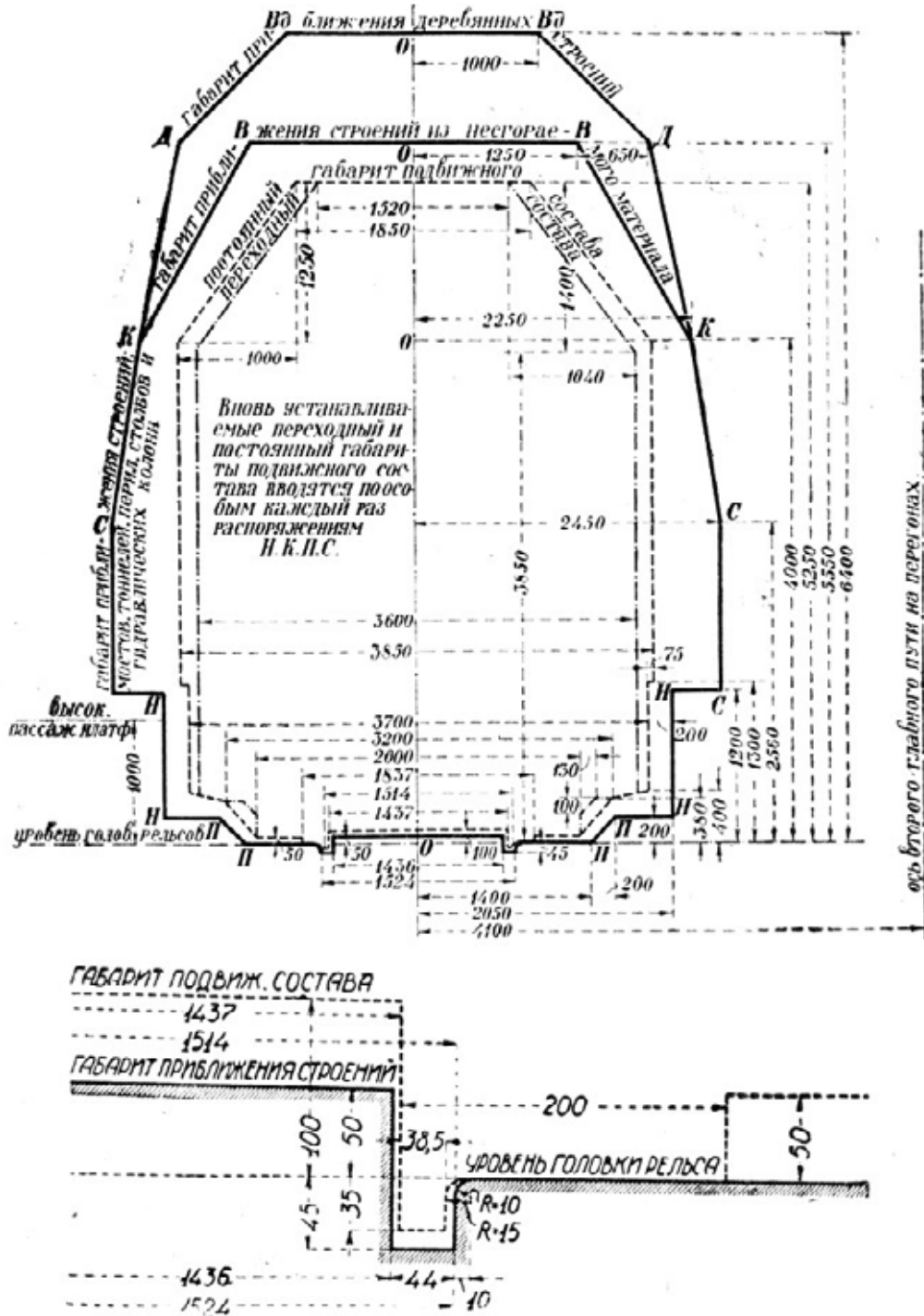
Фиг. 110. Габарит, утвержденный в 1925 г. для применения на всех вновь строящихся железных дорогах, равно при всех капитальных переустройствах.
