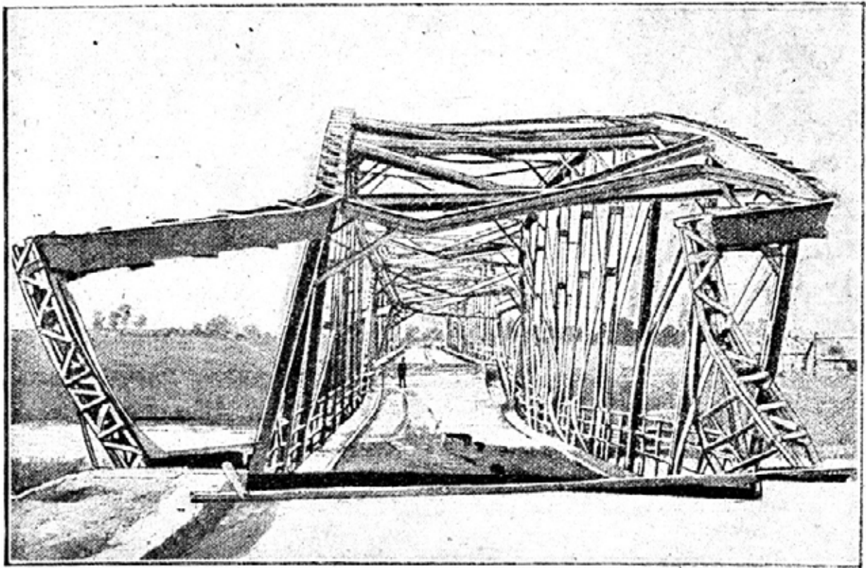
Фиг. 188. Мост, разрушенный при пробной нагрузке.
