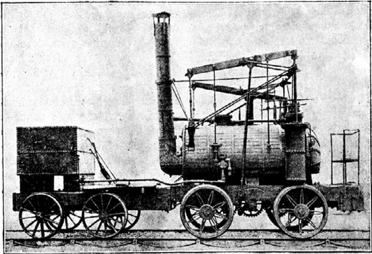
Фиг. 8. Паровоз „Пуффинг Библи”, построенный Хедлеем в 1813 г.
