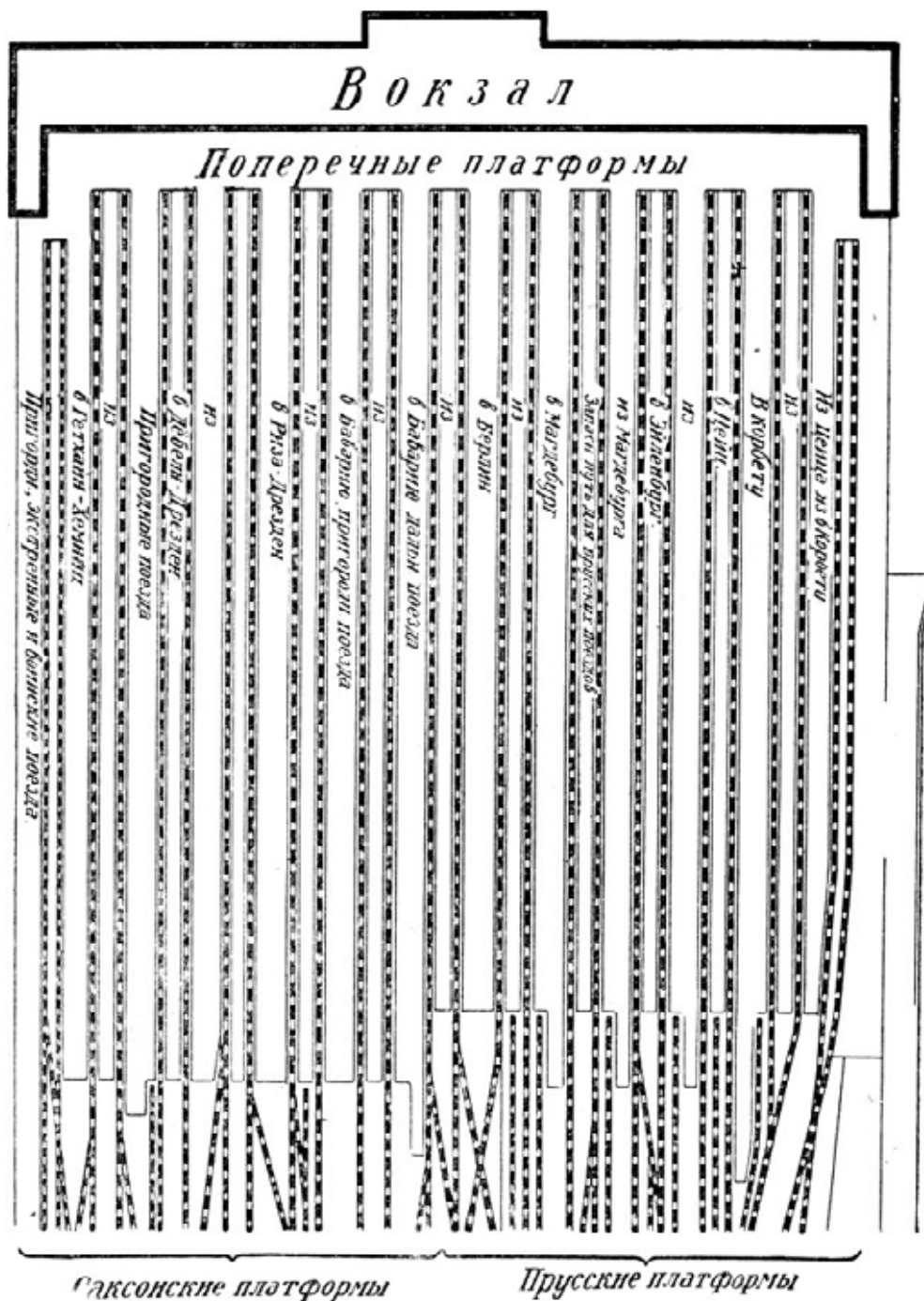
Фиг. 133. Схема станционных путей главного вокзала в Лейпциге.
