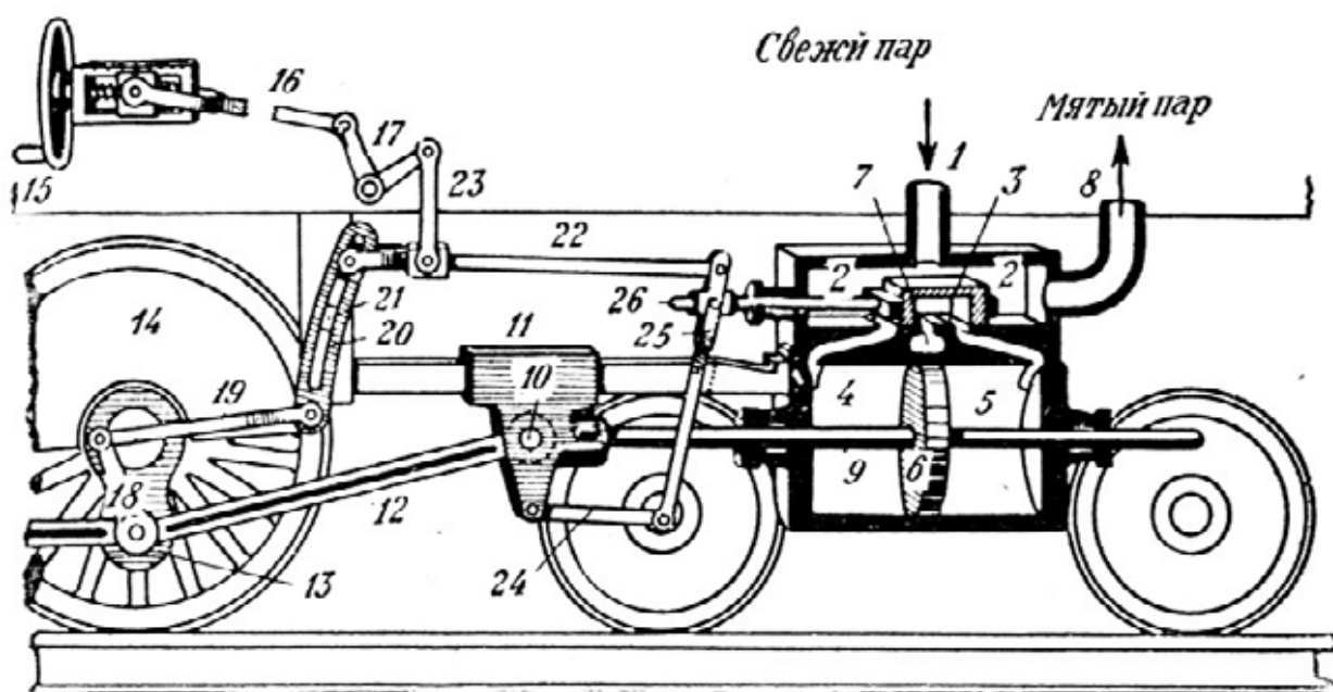
Фиг. 51. Схематическое изображение ходовых частей паровоза.
